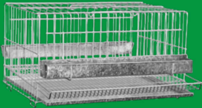
Nº 028B Gaiola Para Codorna Mini Chinesa comp.: 40 cm alt.: 23 cm larg.: 28 cm Opção em Cores: P028B - Zinado Malha entre Arames: 20 mm/ Piso 10 mm Composição.: Arame BTC 1,60 mm x 2,70 mm Capacidade: 10 a 12 Codornas Chinesas Pet Indicado: Codorna Chinesa
