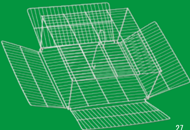
Nº 062 Armadilha para Pesca de Siri comp.: 32cm alt.: 16cm larg.: 32cm Malha entre Arames: 15 mm Opções em Cores: P062 - Zinado E062 - Epóxi Branco
