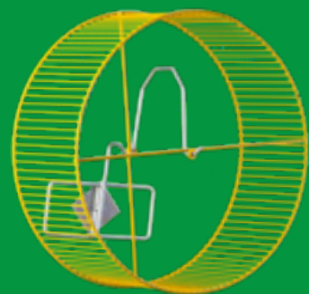
N° 015F Roda Chinchila diâmetro: 30cm larg.: 12,5cm Opções em Cores: Epoxi Malha entre Arames: 9 mm Pet Indicado: Chinchilas
