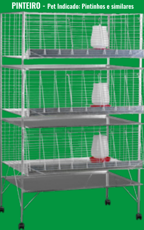
PINTEIRO - Pet Indicado: Pintinhos e similares Nº 033 Com 1 Compart. Fixo comp.: 92cm alt.: 107cm larg.: 70cm Opções em Cores: P033 - Alumínio Nº 033A Com 2 Compart. Fixos comp.: 92cm alt.: 124cm larg.: 70cm Opções em Cores: P033A - Alumínio
