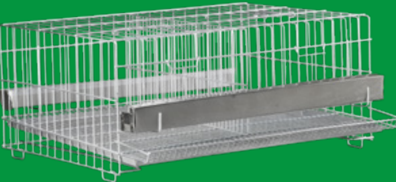
Nº 028A Gaiola para Codorna Nova Poedeira comp.: 50cm alt.: 23cm larg.: 38cm Opções em Cores: P028A - Zinado Malha entre Arames: 25 mm / Piso 10 mm Divisão: 2 Divisórias Capacidade: 18 a 20 Codornas *Obs.: Capacidade para 10 Codornas em cada divisão
