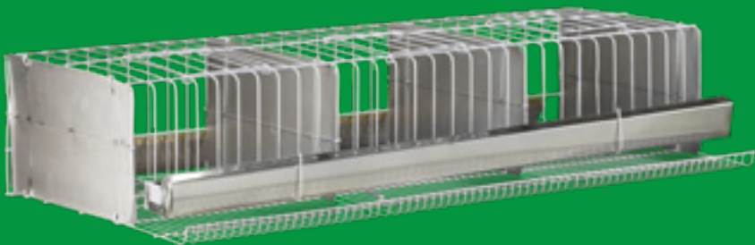
Nº 028A Gaiola para Codorna Nova Poedeira comp.: 50cm alt.: 23cm larg.: 38cm Opções em Cores: P028A - Zinado Malha entre Arames: 25 mm / Piso 10 mm Divisão: 2 Divisórias Capacidade: 18 a 20 Codornas *Obs.: Capacidade para 10 Codornas em cada divisão
