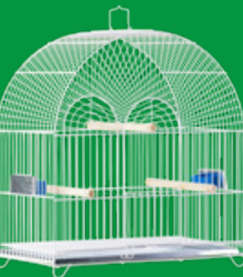
Nº 005RS Gaiola Raio de Sol comp.: 42cm alt.: 43cm larg.: 23cm Opção em Cores: D005RS - Dourado, P005RS - Zincado, E005RS - Epoxi Branco Malha entre Arames: 15 mm
