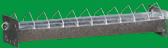
Nº 036 Comedouro Linear 50 cm comp.: 50cm alt.: 10cm larg.: 10cm Malha entre Arames: 47 mm
