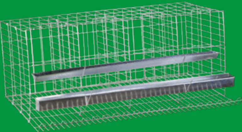
Nº 026 Gaiola para Galinha Poedeira comp.: 100cm alt.: 40cm larg.: 45cm Opções em Cores: P026 - Alumínio Malha entre Arames: 50 mm / Piso 25 mm Divisão: 4 Divisórias Capacidade: 4 a 8 Galinhas *Obs.: Capacidade para 2 galinhas em cada divisão
