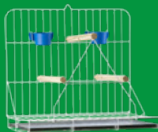
Nº 012A Poleiro Papagaio Dobrável comp.: 49cm alt.: 35cm larg.: 32cm Opção em Cores: D012A - Dourado, P012A - Zincado, E012A - Epoxi Branco Malha entre Arames: 28 mm Pet Indicado: Papagaio manso e similares
