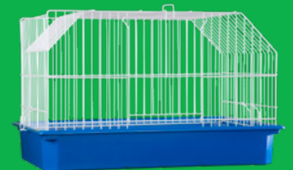
Nº 178 Gaiola Coelho Mini Rex comp.: 54cm alt.: 35cm larg.: 33cm Opção em Cores: P178 - Zincado, E178 - Epoxi Branco Malha entre Arames: 20 mm/ Piso 11 mm *Opção de Pedestal: 092 (Não Acompanha o Produto)
