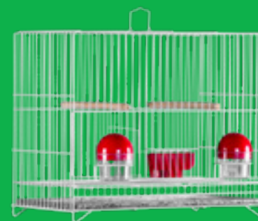
Nº 048 Gaiola Exposição Porte comp.: 40cm alt.: 34cm larg.: 22,5cm Opção Em Cores: P048 - Zincado, E048 - Epoxi Branco Malha entre Arames: 15 mm Padrão porta de Mola na Costa Pet indicado: Exposição de Aves como: Canários, Agapornis, e Outras Aves Exóticas
