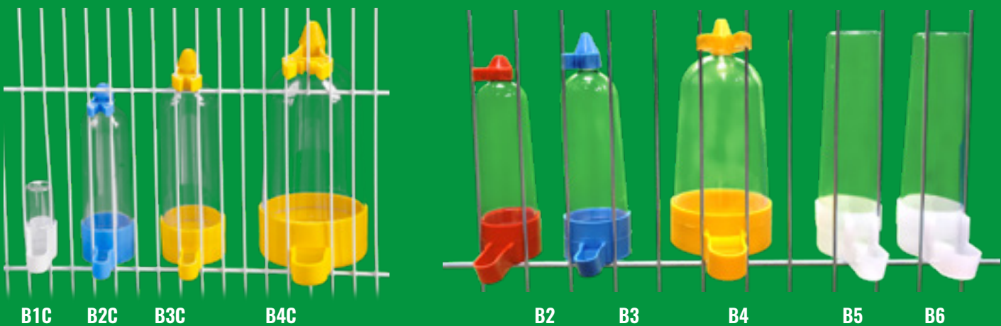
B1C - Mini Bebedouro (Christino) 06 ml B2C - Bebedouro Caçula (Christino) 55 ml B3C - Bebedouro Médio (Christino) 100 ml B4C - Bebedouro Gigante (Christino) 250 ml B2 - Bebedouro Caçula (Pet Fish) 50 ml B3 - Bebedouro Médio (Pet Fish) 65 ml B4 - Bebedouro Gigante (Pet Fish) 200 ml B5 - Bebedouro Profi. (BICO FINO) B6 - Bebedouro Profi. (BICO LARGO)
